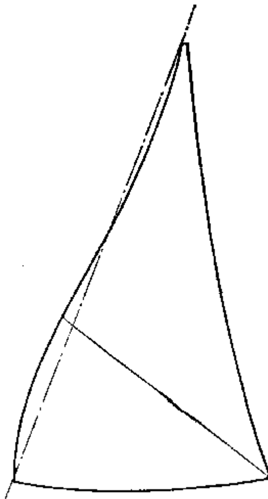
Рис. 6. Раскрой стакселя. Все штаги провисают, поэтому передняя шкаторина стакселя делается криволинейной. Форма этой кривой обеспечивает большую полноту в нижней части стакселя и меньшую — в верхней. Выпуклость нижней шкаторины помогает создать нужную форму
