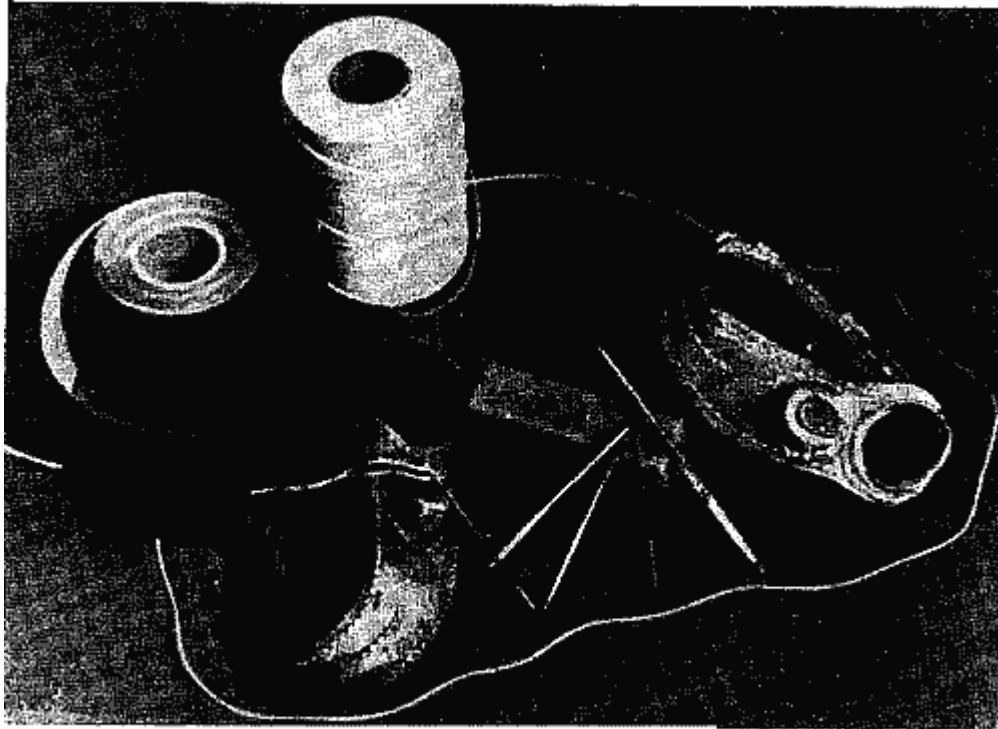
Рис. 51. Оборудование и материалы для парусных работ: слева — моток льняной ленты; сверху — нитки; левый гардаман; для ликовки, правый — для шитья. Между гардаманами — плитка воска и иглы
