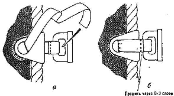
Рис. 22. Крепление ползунков лентой самое надежное, прочное и гибкое. Защитные щитки на ликтросе необязательны (на рисунке показаны пластинчатые щитки)
