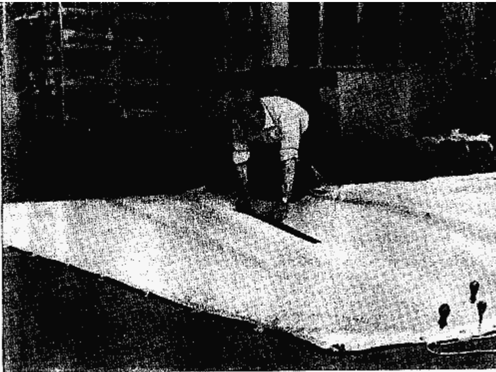
Рис. 43. Увеличение гюта вставкой полотнища
