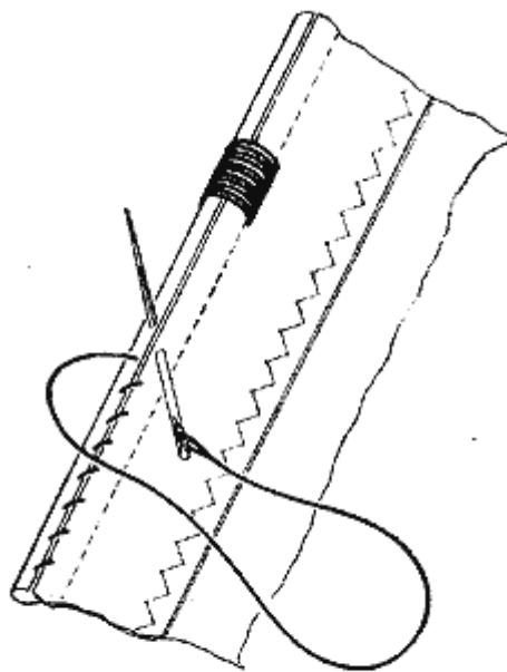
Рис. 20. Ремонт подшивки передней шкаторины: разрезанную подшивку снова зашивают вдоль передней кромки круглым швом
