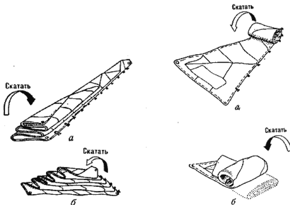
Рис. 14. Складывание стакселя: а — сначала вдоль передней шкаторины; б — потом вдоль нижней, от галсового угла к шкотовому
