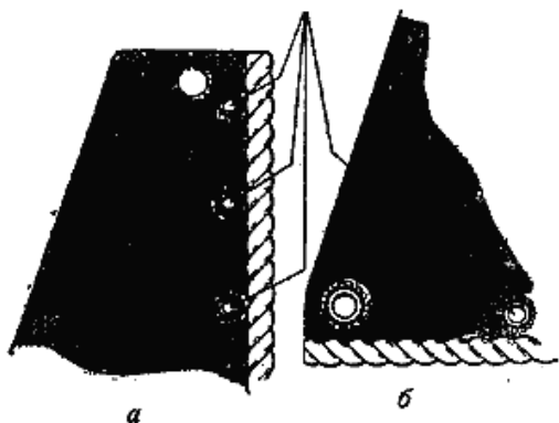
Рис. 49. Переделка грота на крепление ползунками: а — фаловый угол; б — шкотовый угол
