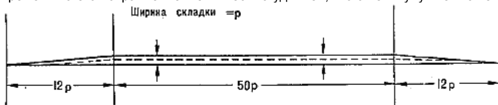
Рис. 38. Относительные размеры складки: постоянная ширина складки должна по длине быть примерно в 50 раз больше, чем полная ее ширина. Законцовки должны быть длиной не менее 12 ширин складки
