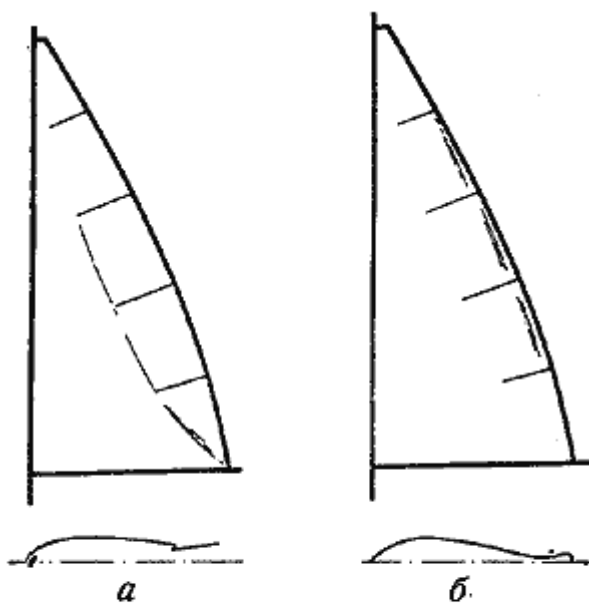
Рис. 33. Растяжение задней шкаторины: а — потянулись и подшивка, и сам парус, образова- лась складка по концам лат; внутренние концы лат на ветру; б — подшивка задней шкаторины натянута туже, чем ткань: «ложка» по задней шкаторине
