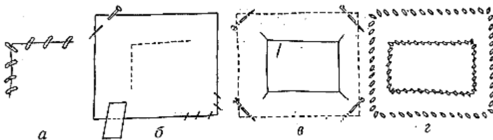
Рис. 64. Постановка заплата
