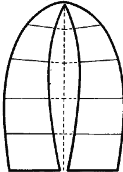
Рис. 46. Уменьшение ширины спинакера
