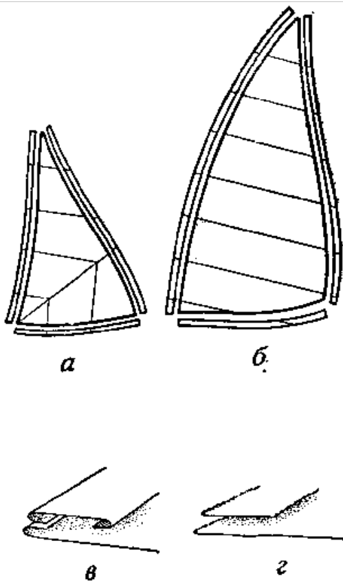
Рис. 11. Отрезная подшивка: a — на стакселе; б — на гроте; в — подшивка с подгибом; г — подшивка с оплавленными кромками
