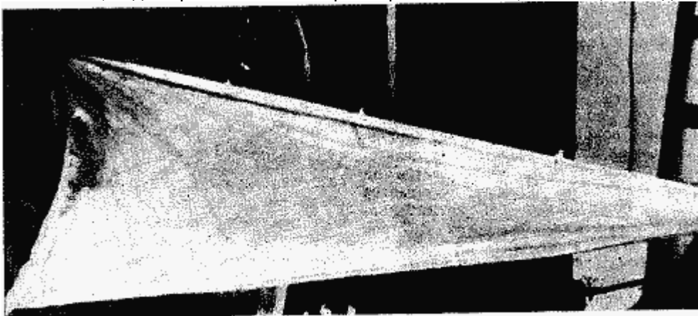
Рис. 35. Прямитивный береговой стенд для проверки формы паруса — парус горизонтально растянут по шкаторинам, ткань свободно провисает и можно проверить его форму
