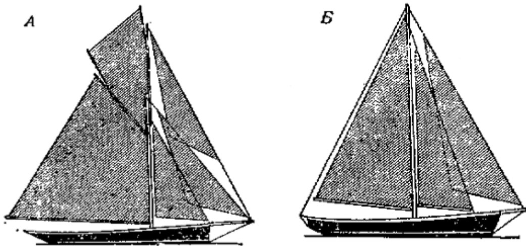
Рис. 14 Тендеры" A — гафельный, Б — бермудский
