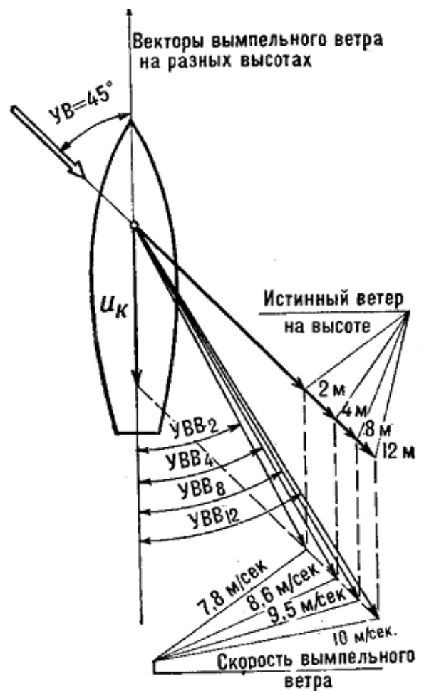
Рис. 93. Изменение вымпельного ветра с высотой
