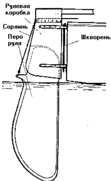
Рис. 32. Устройство подвешного руля швурбота
