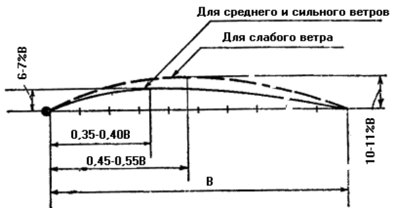
Рис. 96. Профиль паруса
