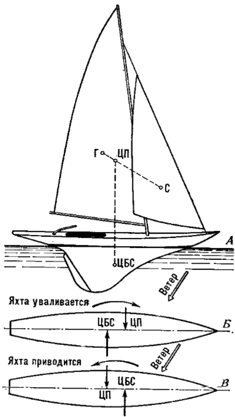
Рис. 99. Центровка яхты
