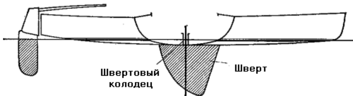
Рис. 5. Швертбот
