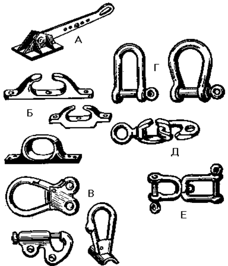
Рис. 51. Дельные вещи:
