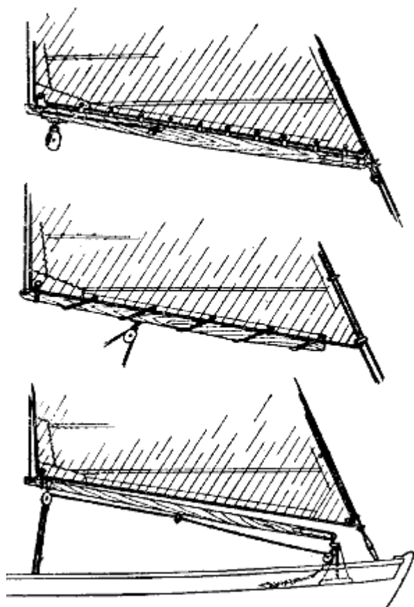
Рис. 43. Рейки стакселей
