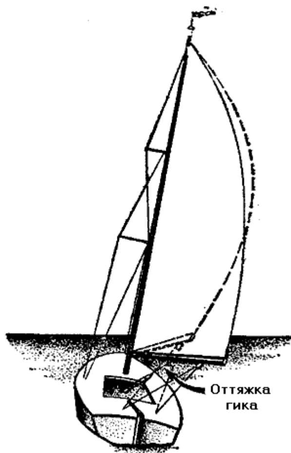
Рис. 112. «Закрутка» гота под ветер
