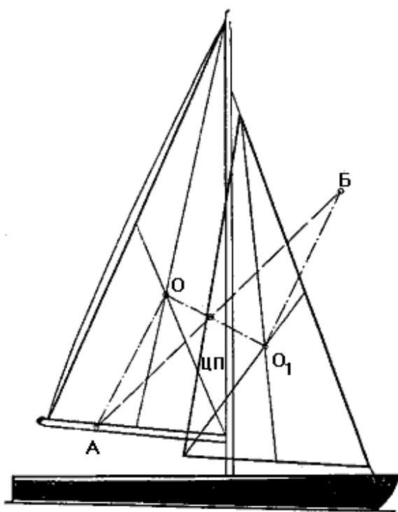
Рис. 98. Графический способ нахождения центра парусности
