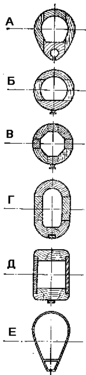
Рис. 37. Сечения рангоута: А — каплевидная деревянная мачта с лик-пазом; Б и В — круглые мачты с рельсами под наружные ползуны; Г и Д — мачты с рельсам под внутренние ползуны, Е — металлическая мачта с лик-пазом
