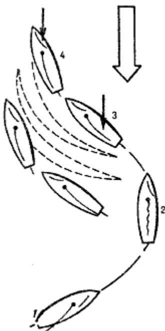
Рис. 120. Яхта в дрейфе
