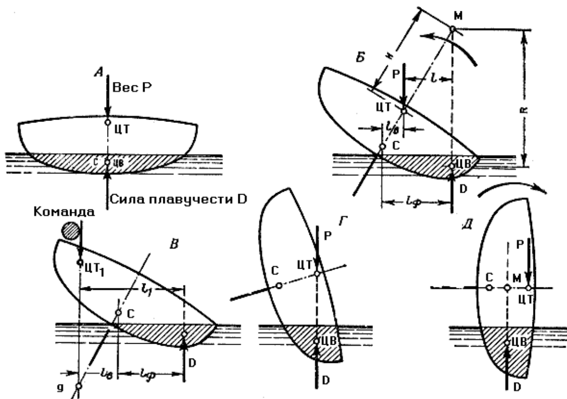
Рис. 78. Остойчивость швертбота
