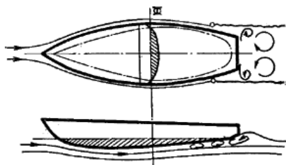
Рис. 84. Образование вихрей у поверхности корпуса яхты
