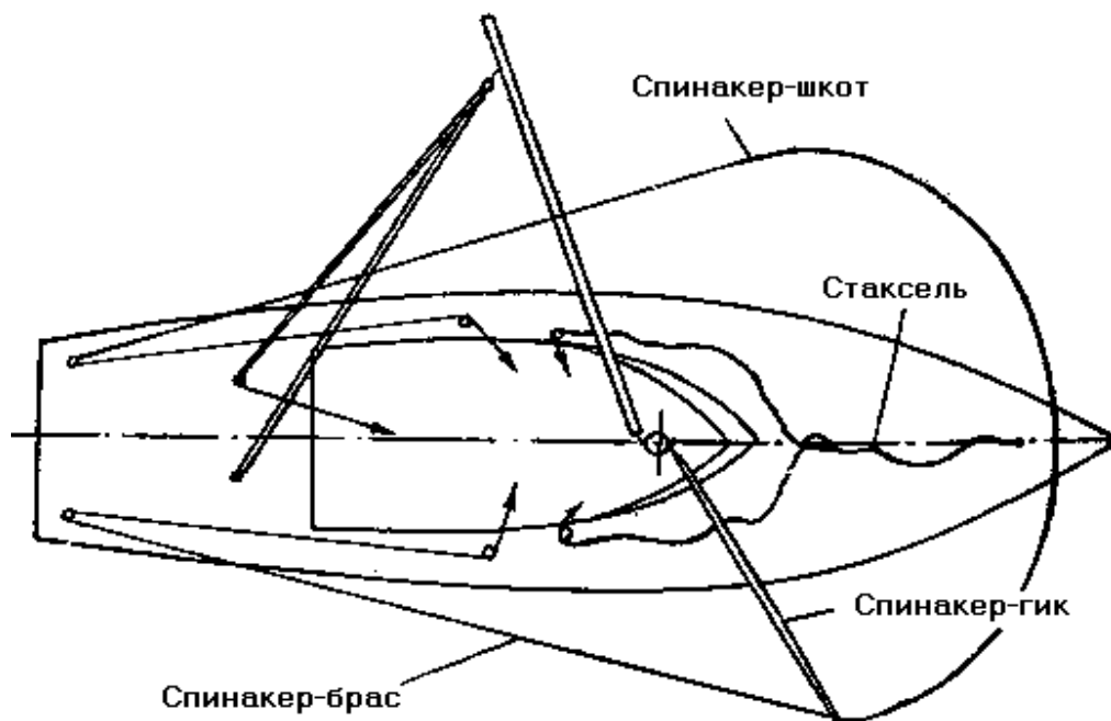
Рис. 48. Такелаж спинакер-гика
