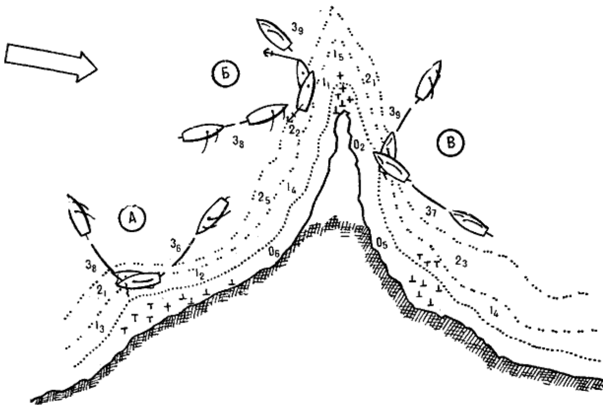
Рис. 138. Случаи посадки на мель: А — на подветренную мель острым курсом; Б — на подветренную мель полным курсом; В — на наветренную мель
