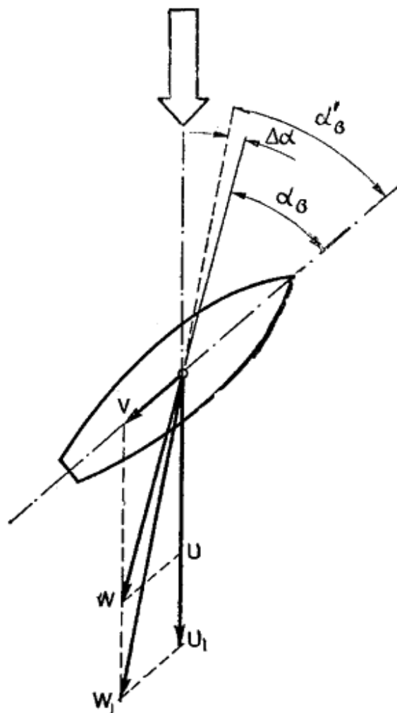
Рис. 92. В полосе сильного ветра можно идти круче
