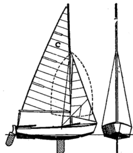
Рис. 22. Гоночная яхта-моготип класса "Солинг"
