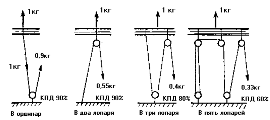
Рис. 44. Некоторые способы проводки гика-шкотов
