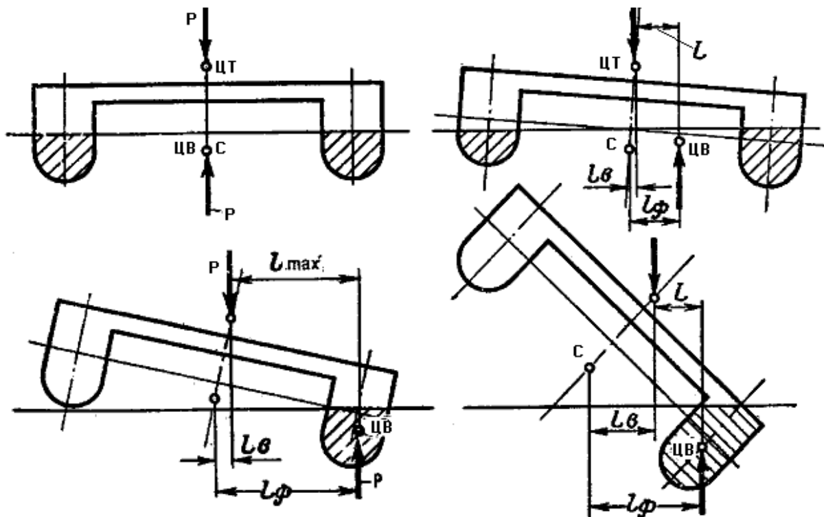
Рис. 81. Остойчивость катамарана
