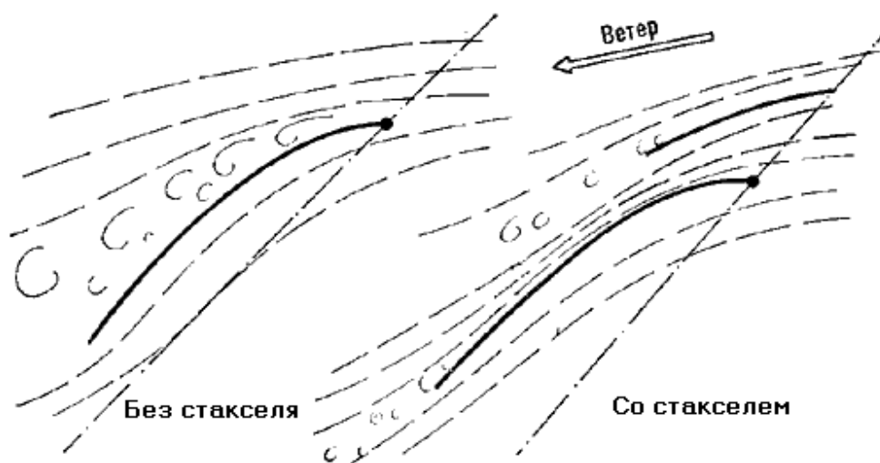
Рис. 97. Работа стакселя
