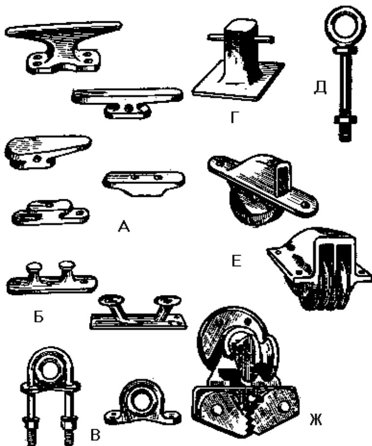
Рис. 50. Дельные вещи: А - утки; Б - кнехты; В - кипы; Г - битенг; Д - обушок; Е - роульсы для проводке такелажа под палубу; Ж - кулачковый стопор
