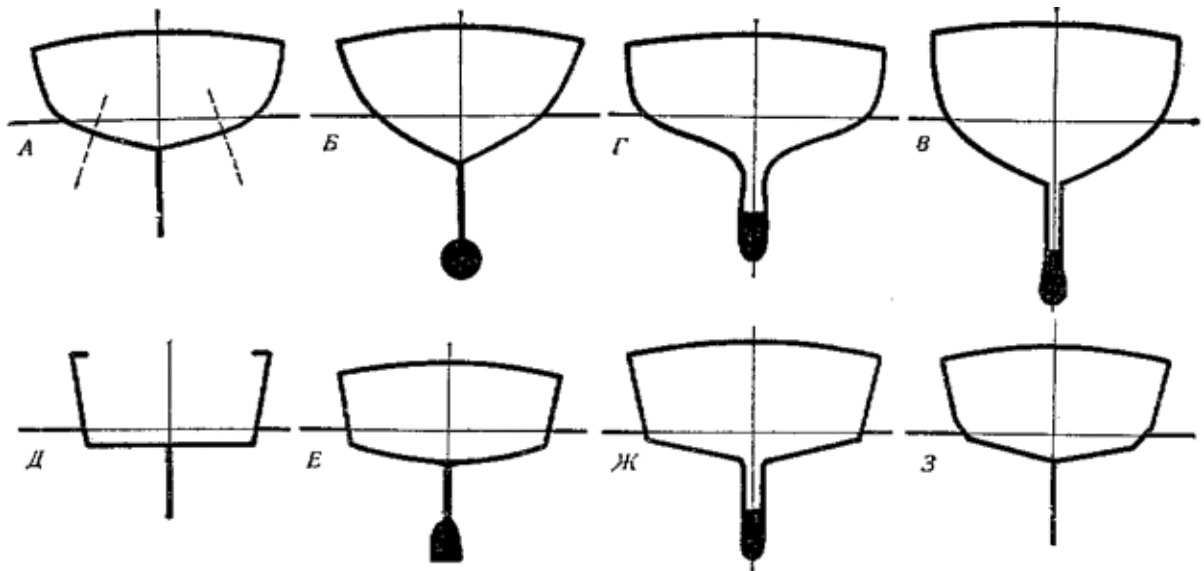
Рис. 9. Формы мидель-шпангоутов.
