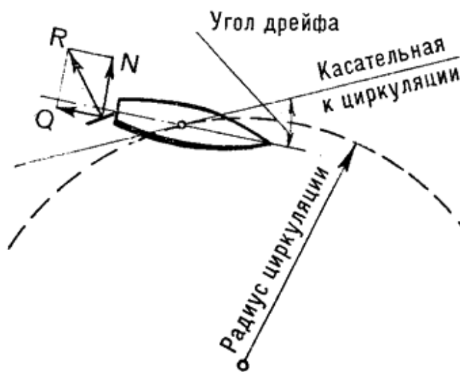
Рис. 83. Схема действия руля
