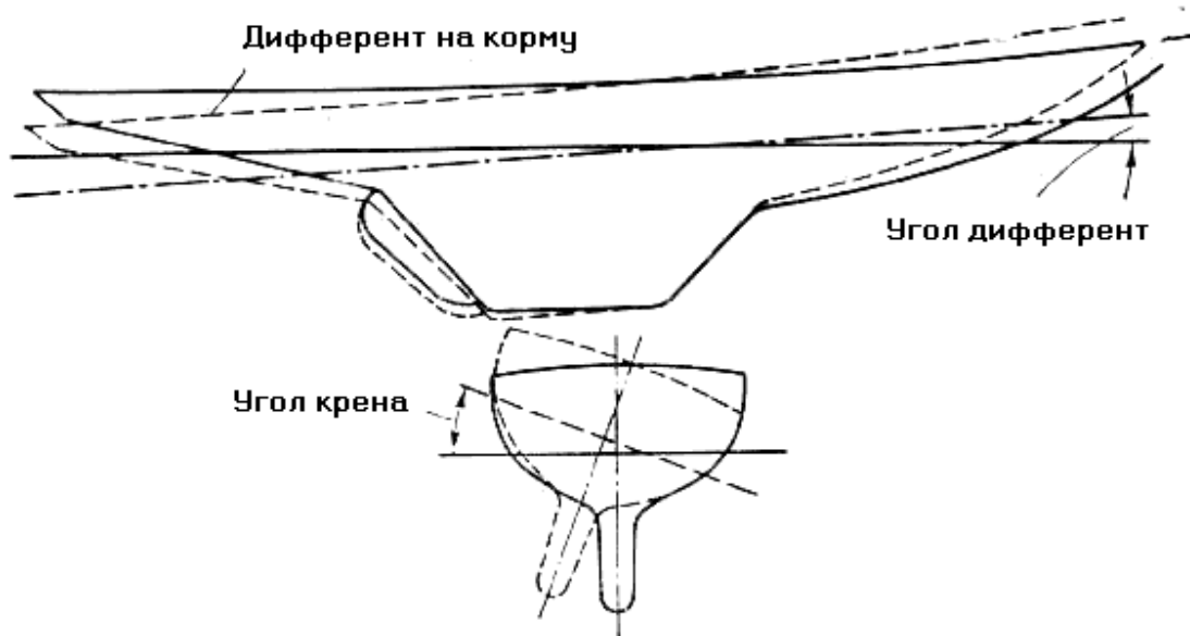
Рис. 77. Крен и дифферент
