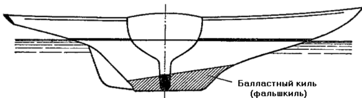
Рис. 4. Килевая яхта
