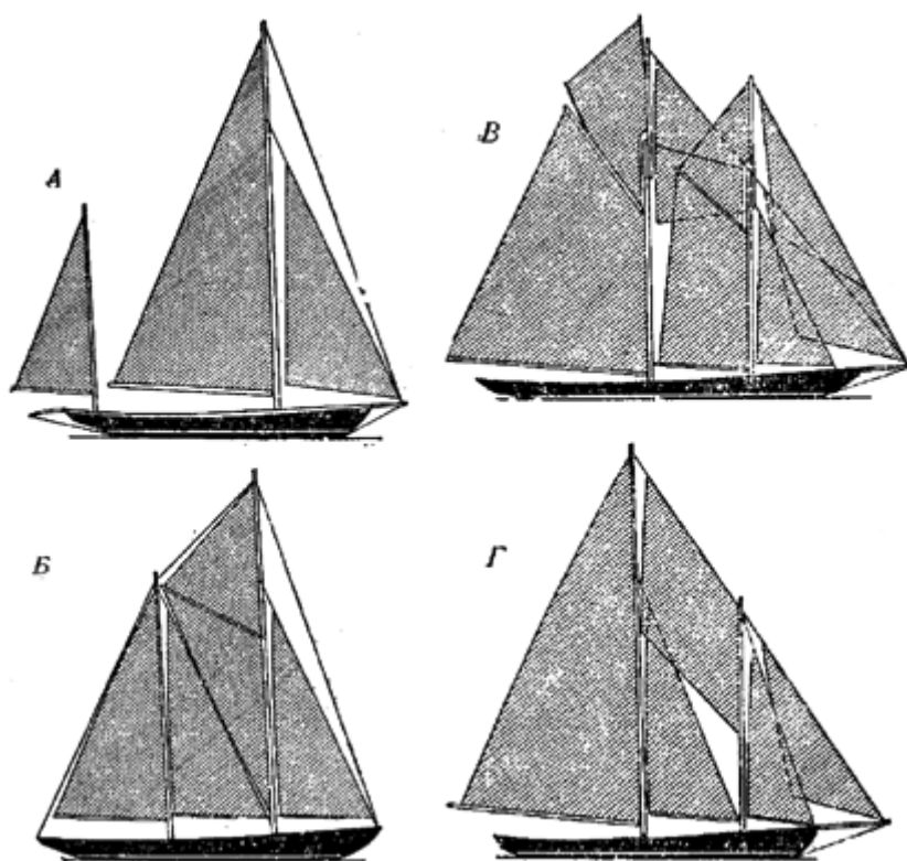
Рис. 15. Двухмачтовые яхты. A — бермудский иол; б — стаксельный кэч. В — гафельная шхуна; Г — бермудская стаксельная шхуна
