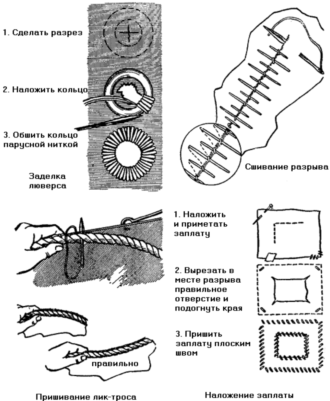
Рис. 72. Ремонт парусов
