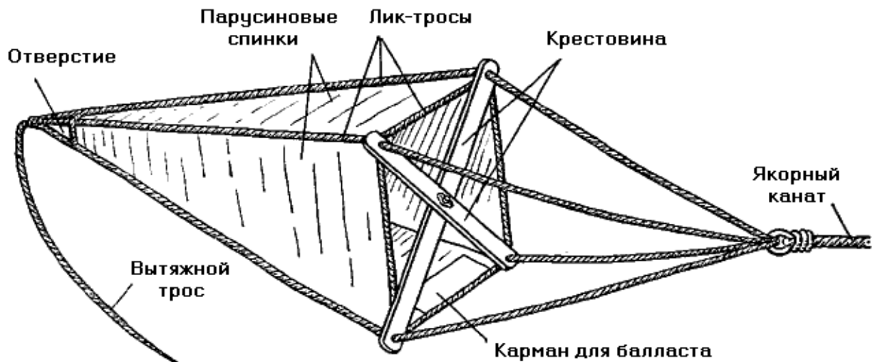
Рис. 117. Плавучий якорь
