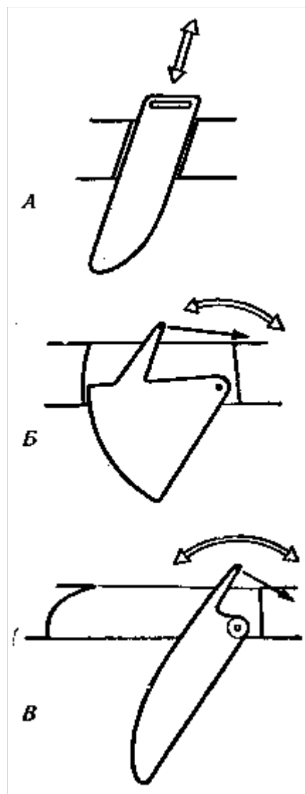
Рис. 33. Типы швертов: А — кинжальный; Б — ющийся секторный, В — качающийся мечевидный
