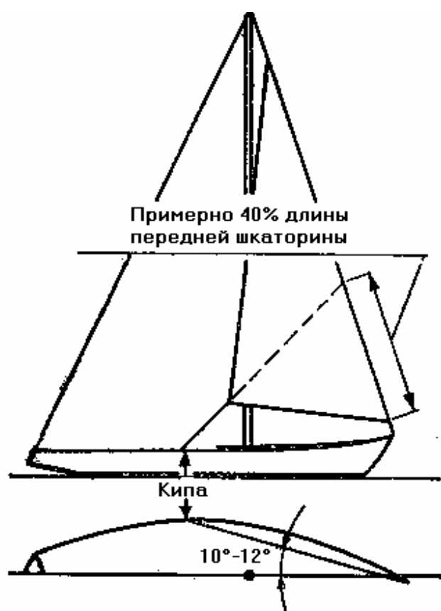
Рис. 46. Проводка стаксель-шкотов
