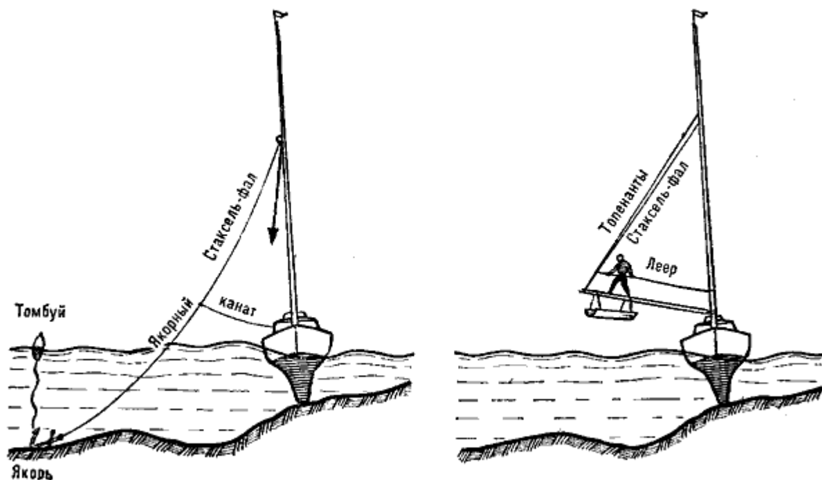
Рис. 139 Способы закрепления яхты на мели
